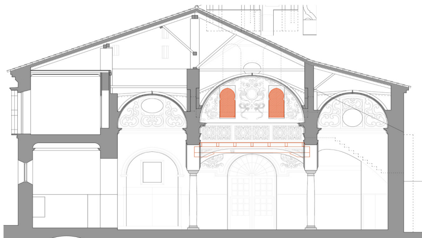
Plano 5. Sección transversal hacia los pies, con las ventanas antiguas restituidas.
